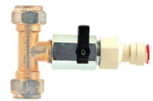
1/2" Male/Male Tee
